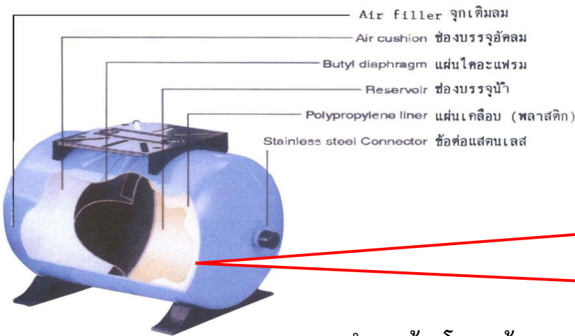
ภาพจำลองด้านโครงสร้างจากรูปแบบถังนอน
